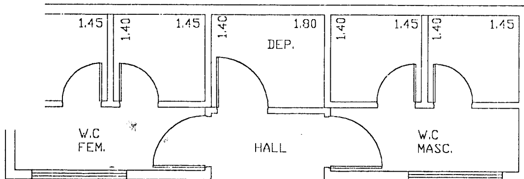
PAVIMENTO INFERIOR
